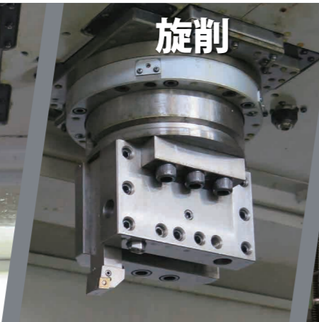
油圧カーボリックランプ
