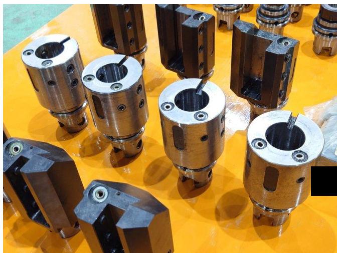
旋盤 ボーリングバーホルダ φ40 3本
